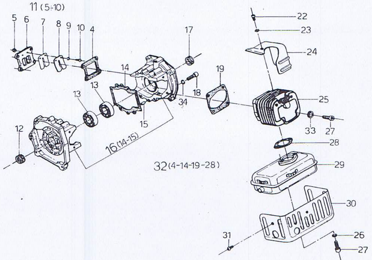
Fig 4 - Engine - Motore
